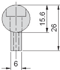
CP-UJT16-8/3030
